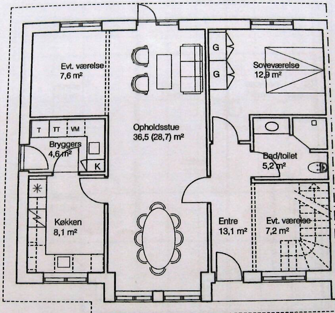
STUEPLAN 95,4 m 2 1:100
